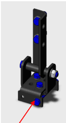
レール貫通ボルト
