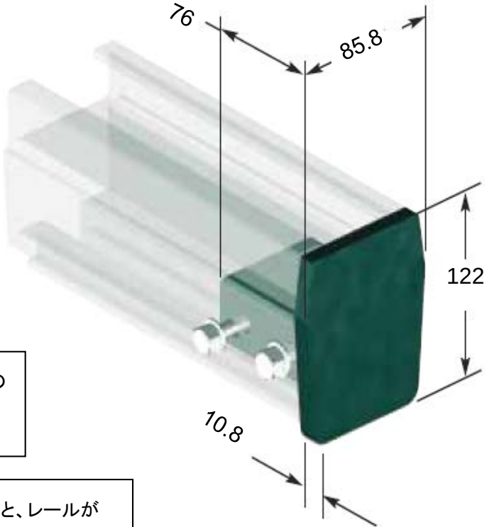
4インチレール寸法
